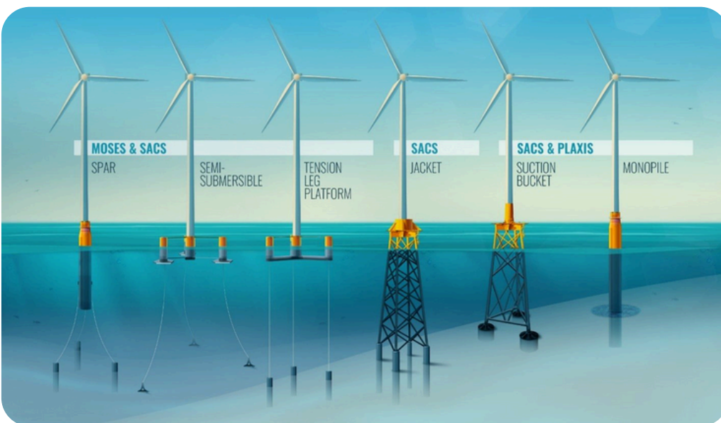
Tuabin gió
